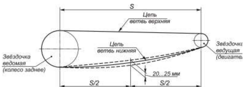
8 – Схема проверки натяжения цепи
